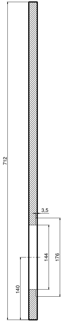
Przekrój płyty bocznej prawej lub lewej
